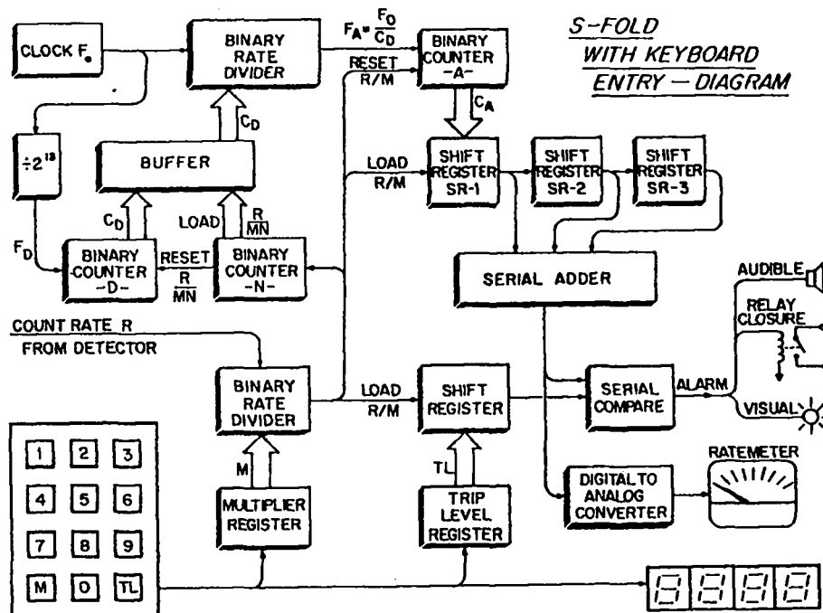
Fig. 3. The s-fold circuit.
